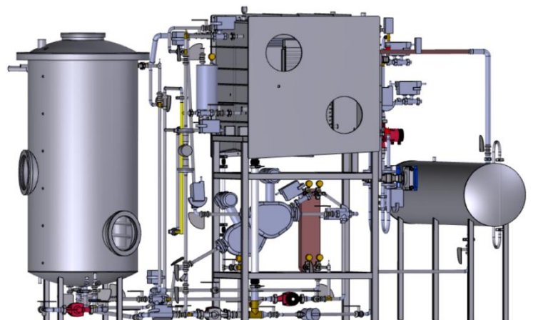
CAD-Modell einer bereits am ZAE Bayern aufgebauten und getesteten Versuchsanlage des Absorptionskältespeichers
