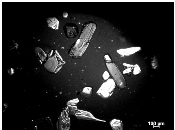
Mikroskopaufnahme von teilweise kristallisierter wässriger Lithiumbromidlösung
